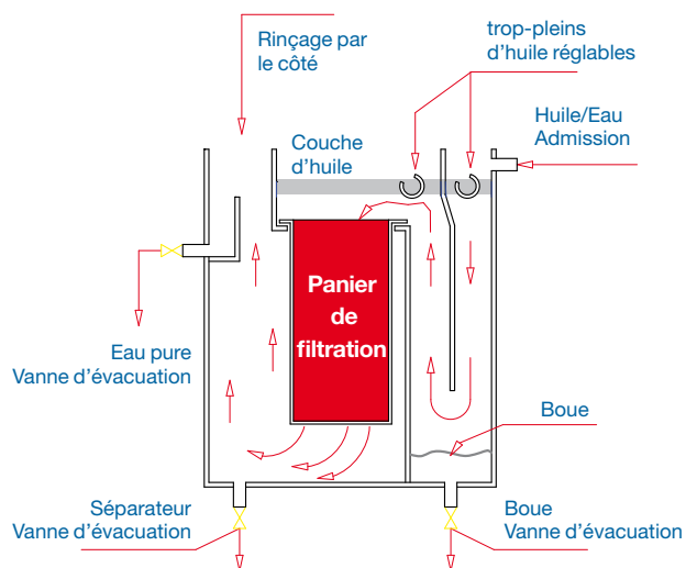
Schéma de fonctionnement LFOS unité d'entretien des émulsions
